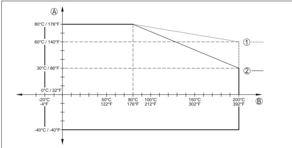
Рис. 39: Температура окружающей среды - температура процесса, исполнение с температурной вставкой
