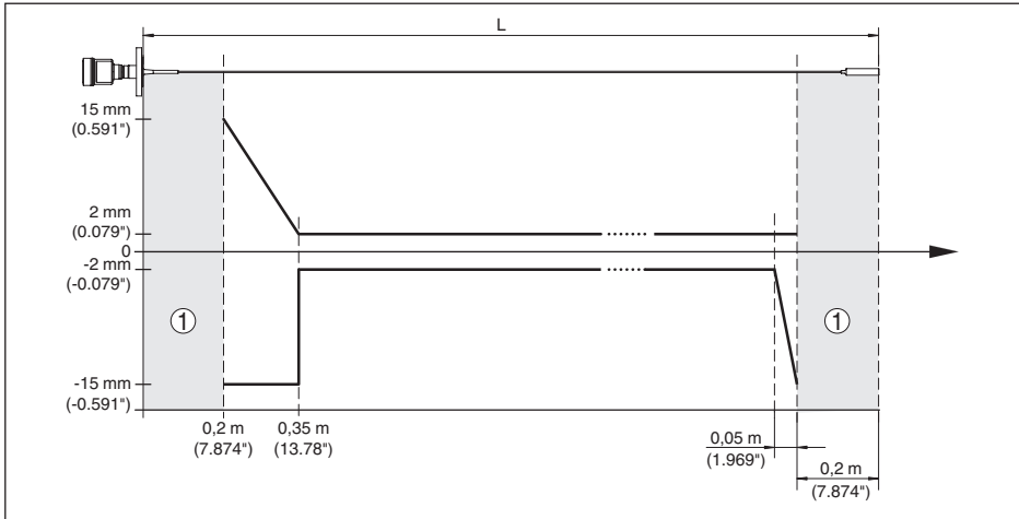
Рис. 37: Погрешность измерения NivoGuide 8100 в тросовом исполнении в 4 мм/0.157 in, с покрытием PFA (среда - масло)
