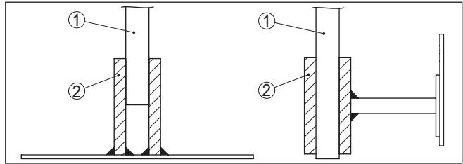
Рис. 9: Фиксация измерительного зонда
