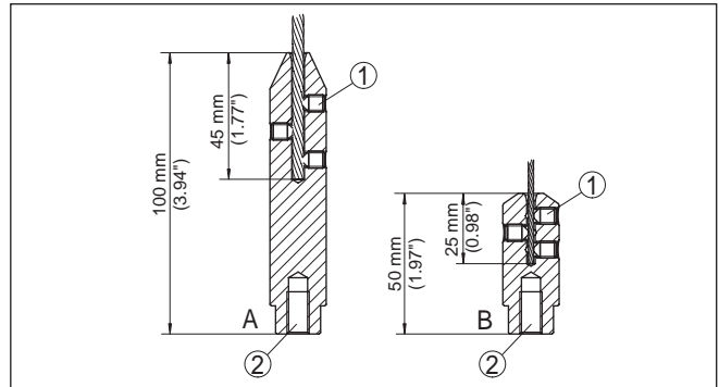
Рис. 29: Укорачивание измерительного троса
