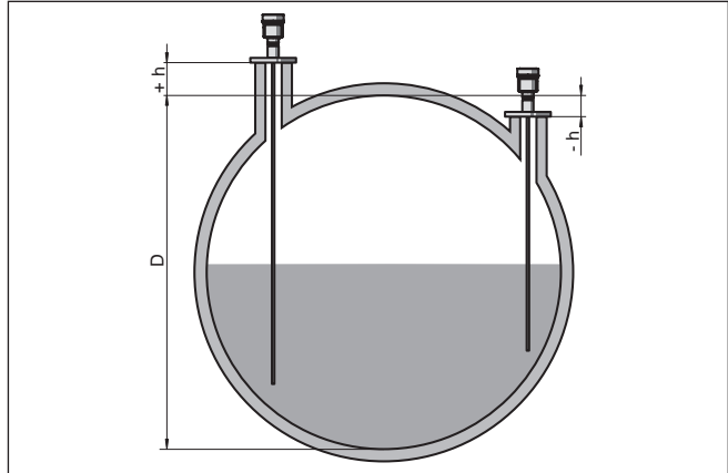
Рис. 17: Высота емкости и значение коррекции патрубка
