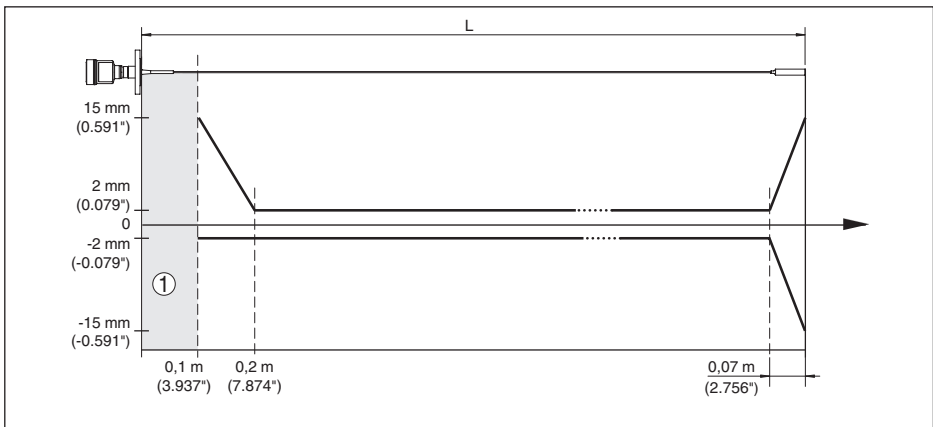
Рис. 36: Погрешность измерения NivoGuide 8100 в тросовом исполнении в 4 мм/0.157 in, с покрытием PFA (среда - вода)
