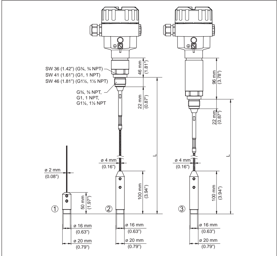
Рис. 42: NivoGuide 8100, резьбовое исполнение с натяжным грузом (все натяжные грузы с резьбой M8 для рым-болта)
