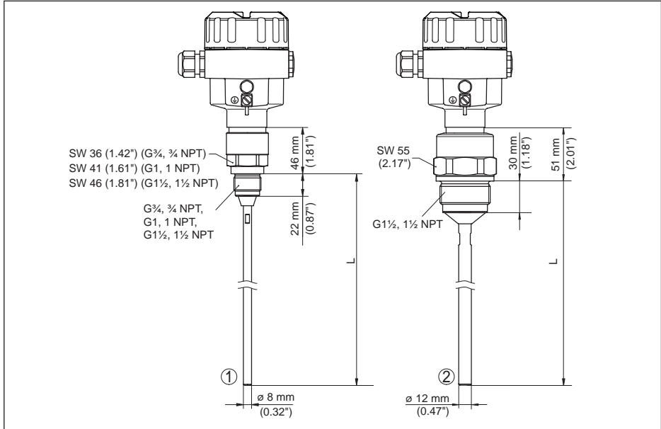
Рис. 43: NivoGuide 8100, резьбовое исполнение
