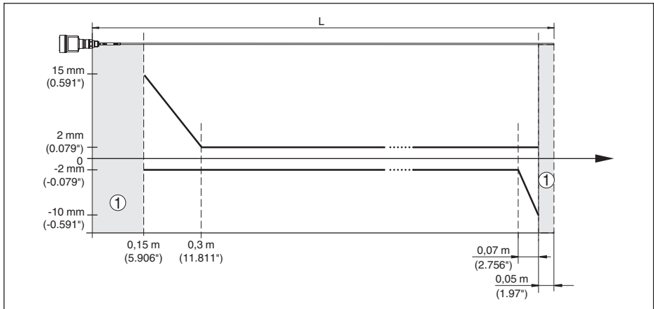
Рис. 32: Погрешность измерения NivoGuide 8100 в стержневом исполнении (среда - масло)
