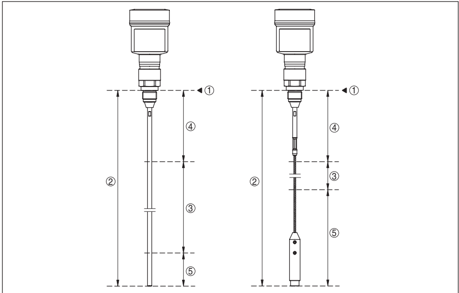
Рис. 30: Диапазоны измерения - NivoGuide 8100
