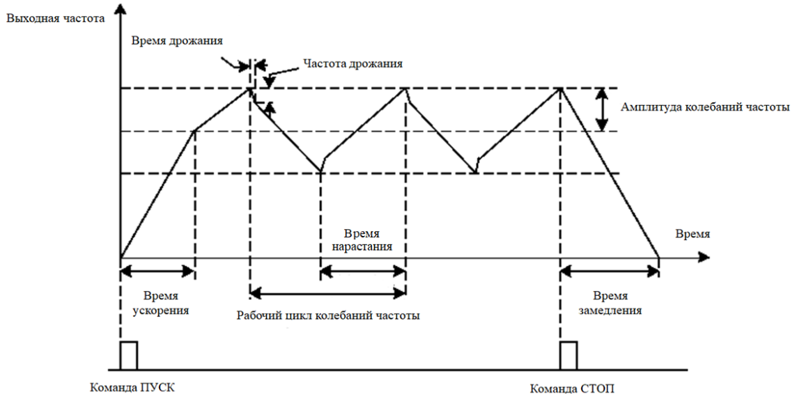
Рис. 6-27 Схема изображения колебаний частоты
