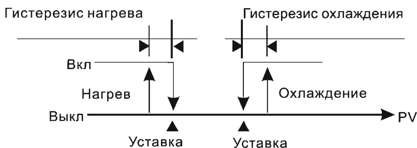
Рис1: Двухпозиционное регулирование для одного выхода
