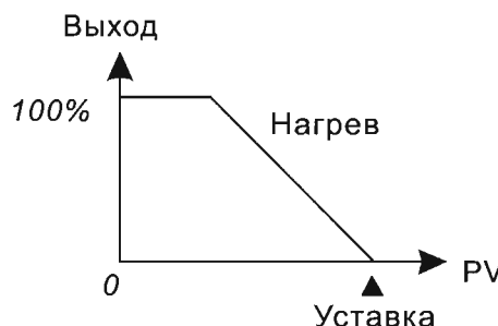
Рис 3: ПИД-регулирование, управление нагревом
