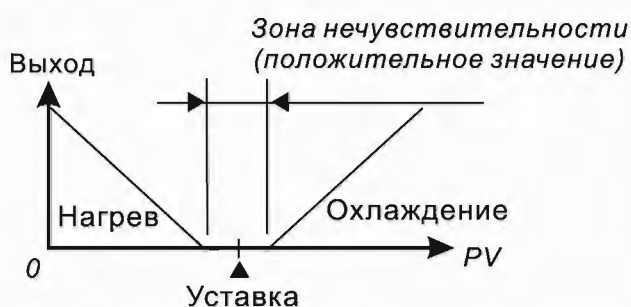
Рис 5: ПИД-регулирование. Двухконтурное управление с положительной зоной нечувствительности
