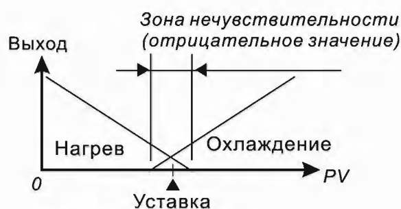
Рис 6: ПИД-регулирование. Двухконтурное управление с отрицательной зоной нечувствительности
