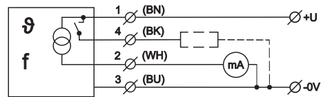
Connection of flow sensor TFS-35_--_--IFPP and TFS-35_--_--IFPT
