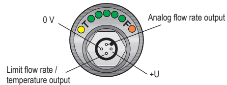
Connector of flow sensor TFS-35_--_--IFPP and TFS-35_--_--IFPT
