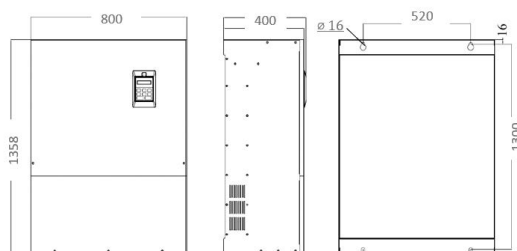
Рис. 1-13. Габаритные размеры преобразователей частоты с мощностью от 315 кВт до 400 кВт
