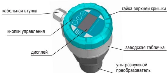
Рис. 23: Описание главных частей измерителя уровня
