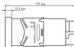
Вид сбоку
