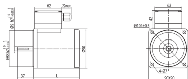
Электродвигатель 40 Вт L=105 мм
