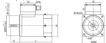
Электродвигатель 60 Вт L=128 мм, 90 Вт L=142 мм
