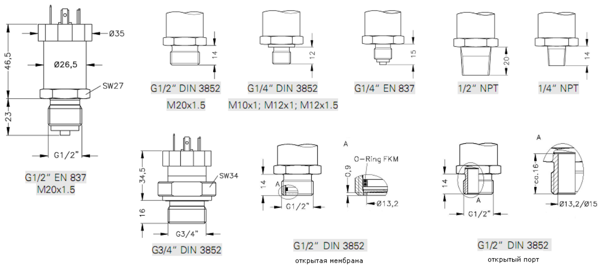
Рисунок Б.4 – Габаритные размеры и размеры различных типов механических присоединений датчиков давления DMP 457
