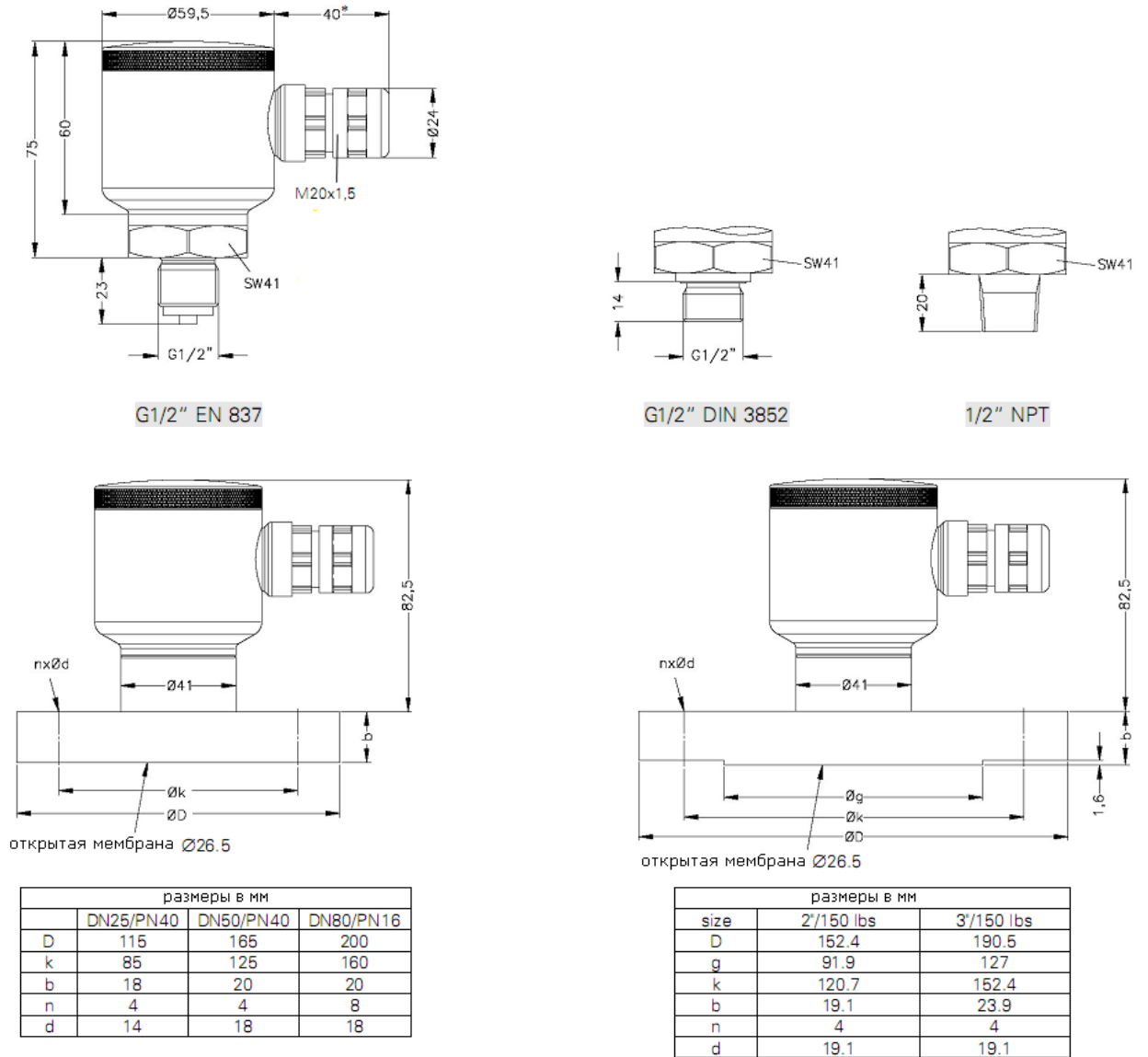
Рисунок Б.1 – Габаритные размеры и размеры различных типов механических соединений датчика давления DMK 456.
