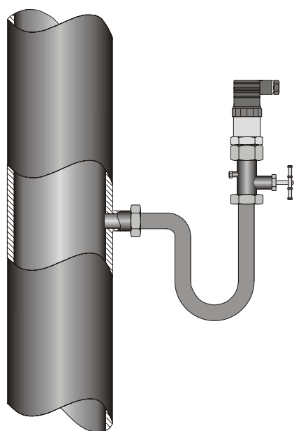
Рисунок 1. Монтаж датчика для измерения давления газа.
