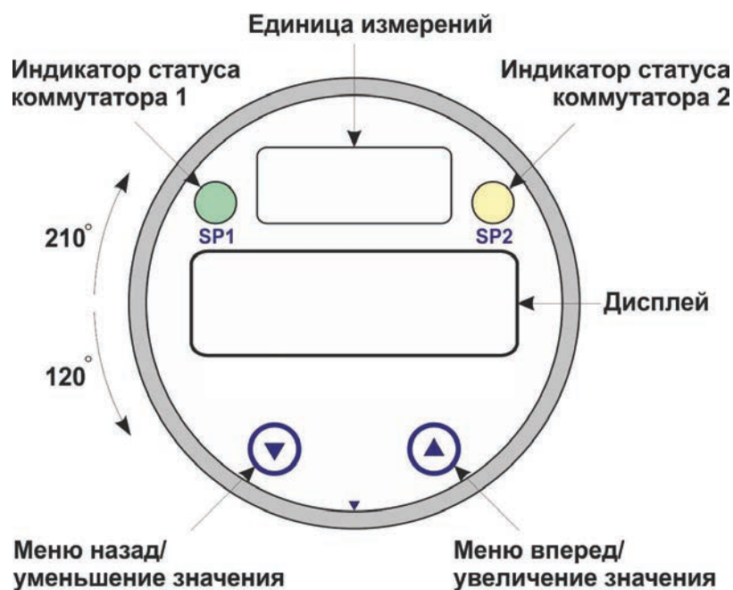
Рисунок 3.1 – Внешний вид панели индикации и управления прибора
