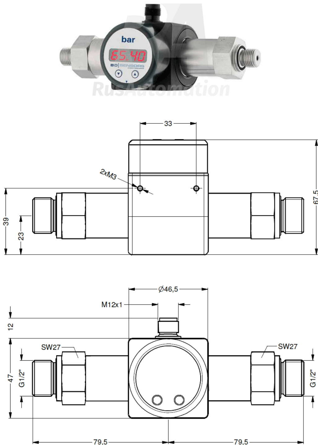
Рисунок Б.1 – Габаритные размеры корпуса прибора
