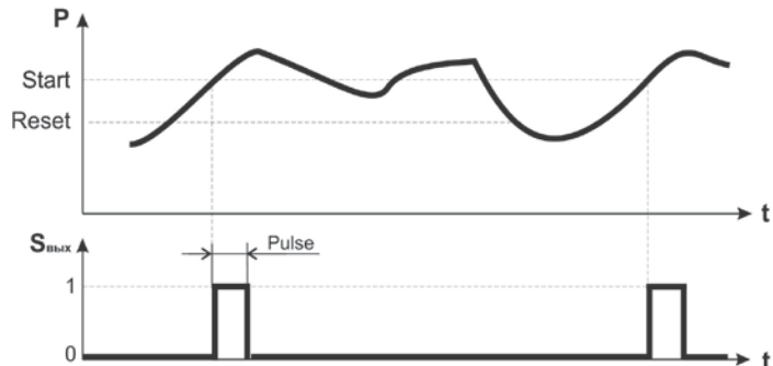
Рисунок 6 – Прямой режимы работы коммутационных выходов (S вых ) при изменении входного давления (P)
