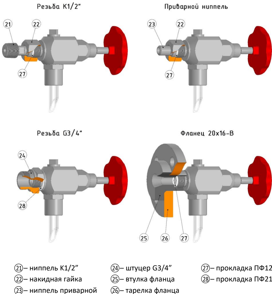
Рисунок 7.2.2 – Устройство указателя уровня с опциональными присоединениями (остальное – см. рисунок 7.2.1)
