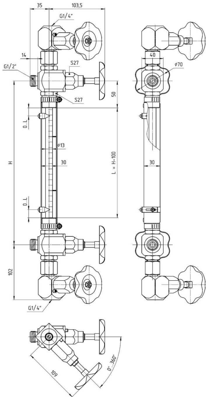
Рисунок 7.1.1 – Общий вид указателя с присоединительной длиной H \leq 1500 мм и резьбовым присоединением G1/2"
