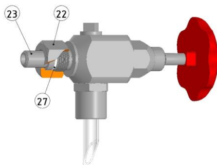
Приварной ниппель
