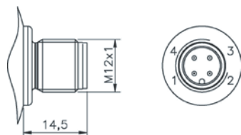
M12X1 (4 конт.)
