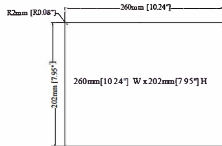
Cutout Dimensions
