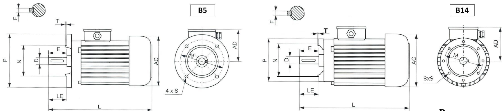
Размеры, мм
